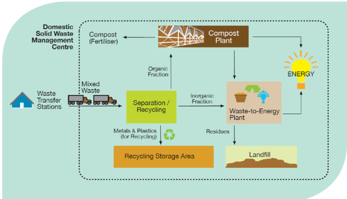
رسم يشرح كيفية عمل المنشأة في قطر
